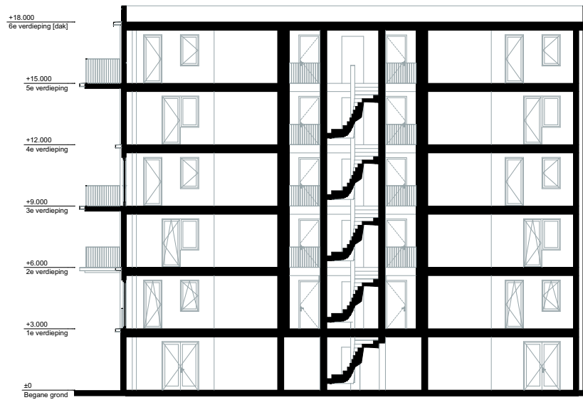
Doorsnede A
