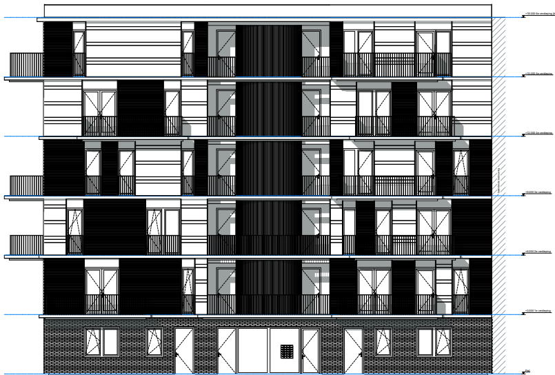
Noordgevel
