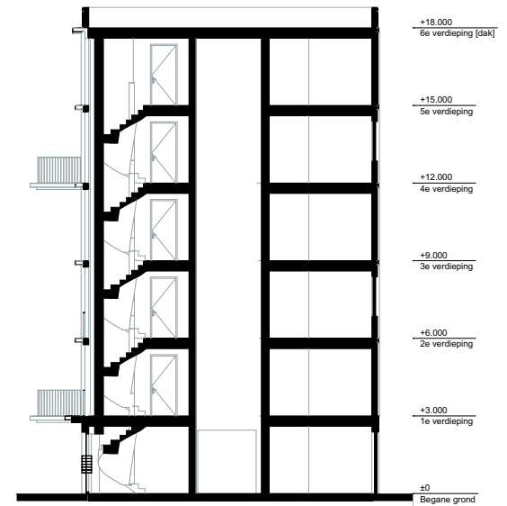
Doorsnede C
